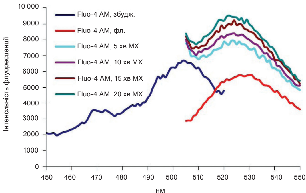
Рис. 2. Спектри збудження та флуоресценції \text{Ca}^{2+} -чутливого флуоресцентного зонда Fluo-4 АМ у контролі та в умовах його взаємодії із МХ міометрія в часі
