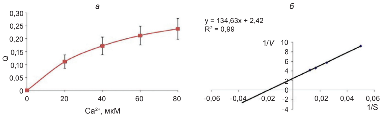
Рис. 5. Акумуляція \text{Ca}^{2+} енергізованими МХ міометрія в залежності від концентрації \text{Ca}^{2+} в робочому середовищі, M \pm t ; n = 5 (а). Приклад типового розрахунку (б) константи активації акумуляції \text{Ca}^{2+} в МХ міометрія (координати Лайнуївера–Берка), де 1/V = F_0/F - F_0 за 1 \text{ хв}^{-1}
