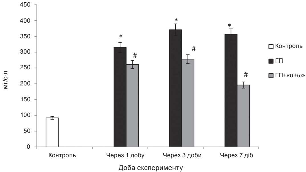
Рис. 1. Активність α-амілази в плазмі крові щурів за гострого панкреатиту та за введення БАД «Альфа+омега» ( M \pm m, n = 5 ): контроль – 1 група; через 1 добу: 2 група – тварини з ГП, 3 група – тварини з ГП +«α+ω»; через 3 доби: 4 група – тварини з ГП, 5 група – тварини з ГП + «α+ω»; через 7 діб: 6 група – тварини з ГП, 7 група – тварини з ГП +«α+ω»; * вірогідність відмінностей порівняно з контролем, P < 0,05 ; # вірогідність відмінностей порівняно з тваринами з ГП відповідних термінів, P < 0,05
