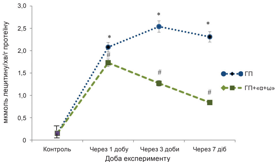
Рис. 7. Активність ФЛА 2 у плазмі крові щурів за гострого панкреатиту та за введення БАД «Альфа+омега», ( M \pm m , n = 5 ), * відмінності вірогідні порівняно з контролем, P < 0,05 ; # відмінності вірогідні порівняно з тваринами з ГП відповідних термінів, P < 0,05
