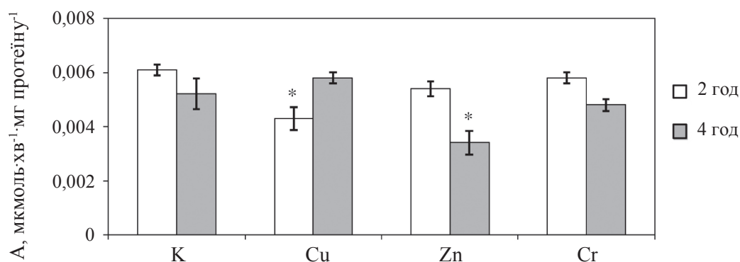
Рис. 6. Активність АОХ (мкмоль·хв -1 ·мг протейіну -1 ) в репортерного штаму CBS4732 prGSH2-AOX дріжджів H. polymorpha за вирощування у середовищі YNB з 3%-ю глюкозою без (К) та з іонами міді, цинку або хрому в концентрації 25 мкМ; * P < 0,05 у порівнянні з відповідним контролем
