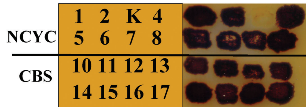
Рис. 3. Якісне визначення активності АОХ у клітинах дріжджів, вирощених на багатому середовищі YPD. Буквою К позначений штам дикого типу NCYC495 leu1-1 , а цифрами – штамми, що містять репортерну касету prGSH2-AOX
