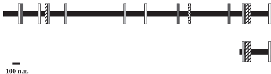
Рис. 2. Схема молекулярної організації 5'-фланкуючої ділянки гену GSH2 H. polymorpha розміром 3712 і 450 п.н. Ймовірні сайти зв'язування транскрипційних факторів такі як позначено на рис. 1
