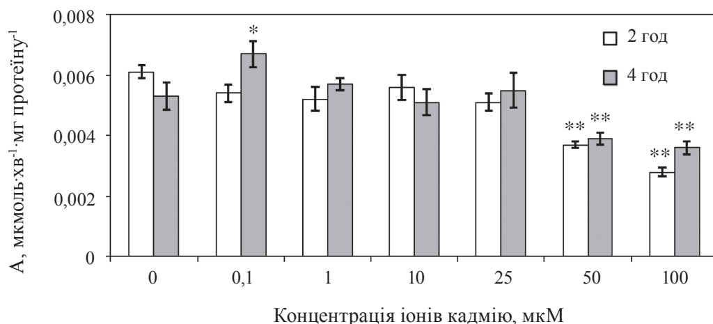
Рис. 5. Активність АОХ (мкмоль·хв -1 ·мг протейіну -1 ) в репортерного штаму CBS4732 prGSH2-AOX дріжджів H. polymorpha за вирощування в середовищі YNB з 3%-ю глюкозою за присутності різних концентрацій іонів кадмію; * P < 0,05 , ** P < 0,005 у порівнянні з відповідним контролем; кореляційний аналіз між концентрацією іонів кадмію та активністю АОХ на другу ( P < 0,005 ; коеф. кореляції -0,960 ) та четверту ( P < 0,05 ; коеф. кореляції -0,873 ) годину інкубації
