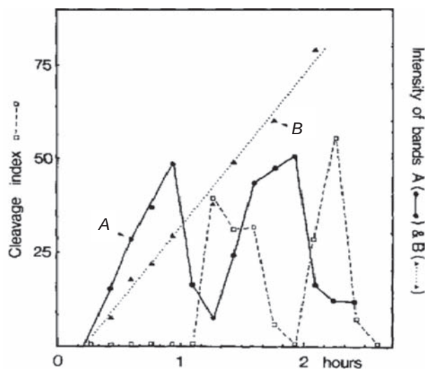
Рис. 5. Кореляція рівня цикліну з циклом поділу клітини: циклін А (●—●); протеїн В (▲···▲); індекс поділу (□--□) [26]
