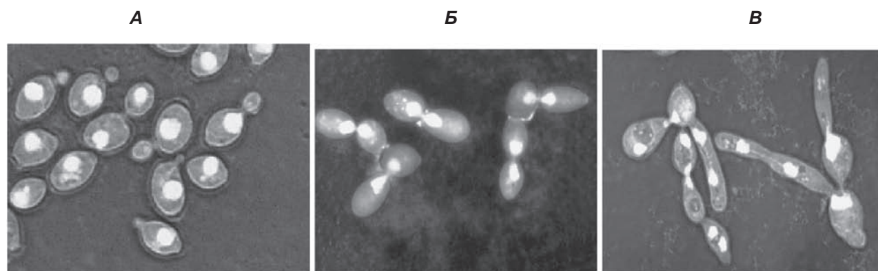
Рис. 2. Нормальні дріжджеві клітини Saccharomyces cerevisiae та cdc мутанти через декілька годин після інкубації за обмежувальної температури. (А) дикий тип (Б) cdc8 , (В) cdc10 [7]
