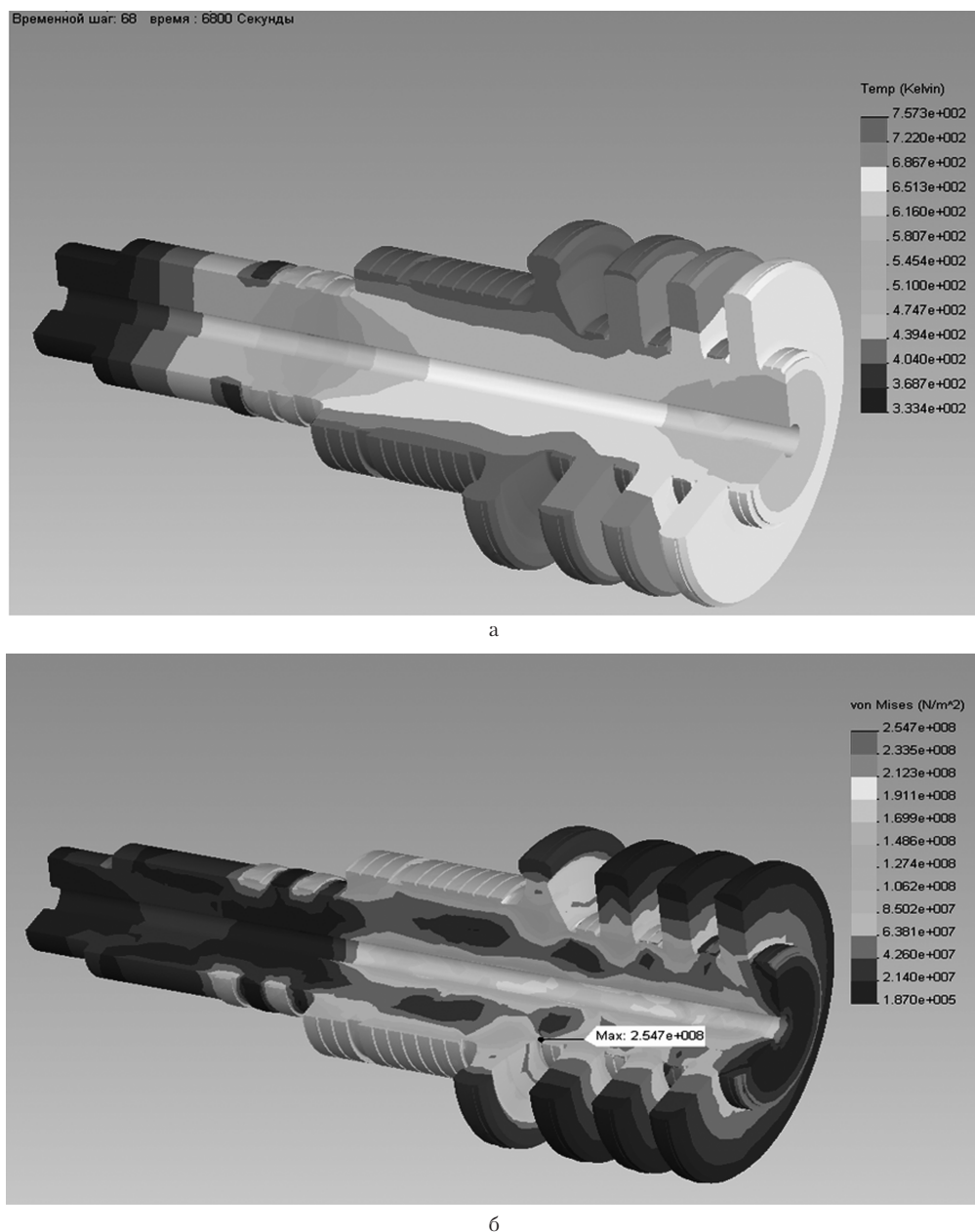
Рис.3. ТС (а) и НДС (б) для РСД при пуске из НС-2 в момент времени 6800 с.
