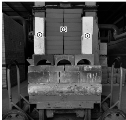
Рис.1. Вариант садки огнеупорных изделий с муфелем: 1 — муфель; 2 — пакет изделий.
