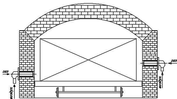
Рис.3. Схема расположения горелок в стенах печи.
