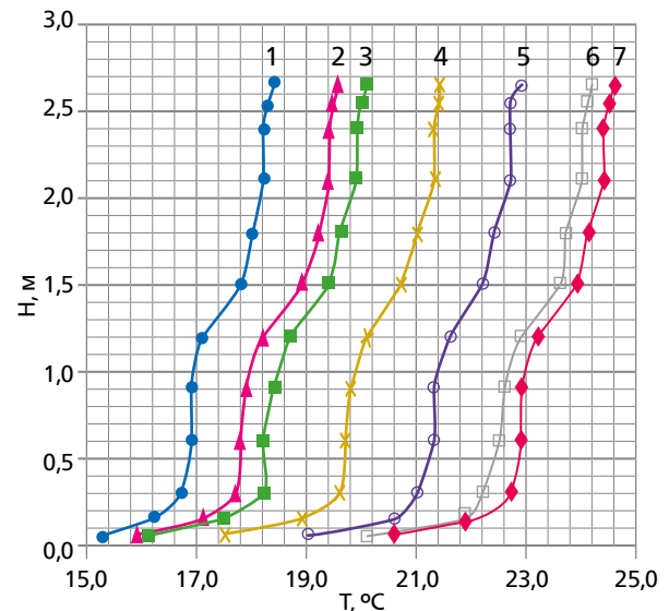
Рис. 7. Зміна профілю температури при нагріванні приміщення електричними керамічними нагрівачами:
