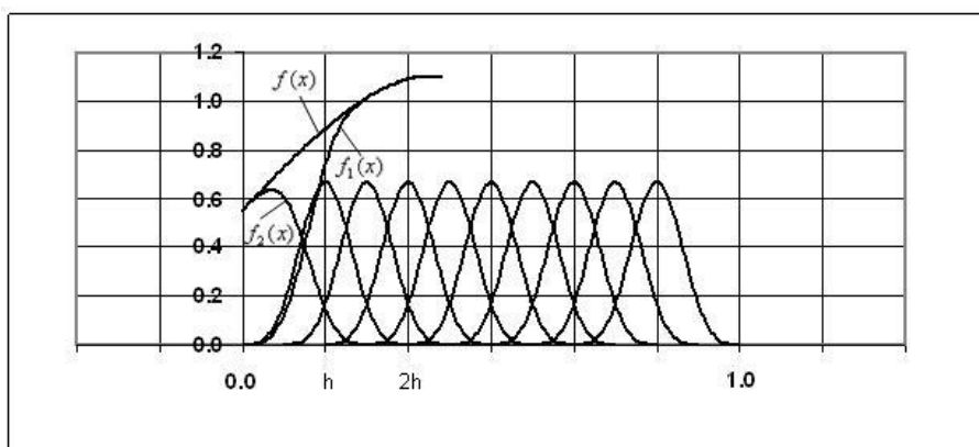
РИС. 3. Функции f_1(x) и f_2(x)
