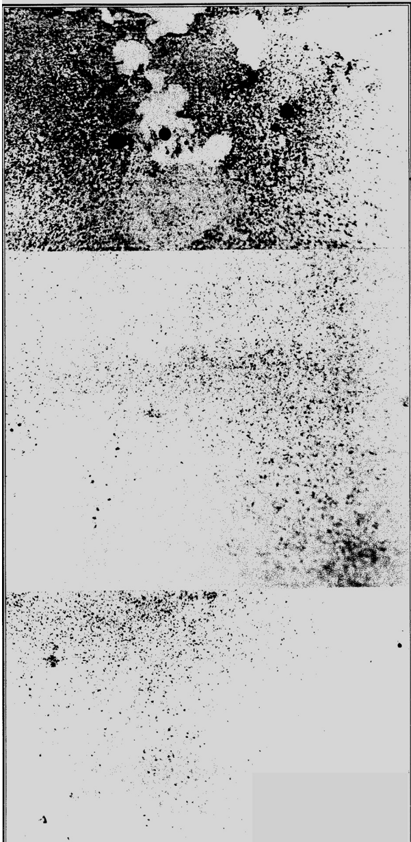
Рис. 2. Отпечаток по Бауману слитка из булатной стали с содержанием 0,022 % S
