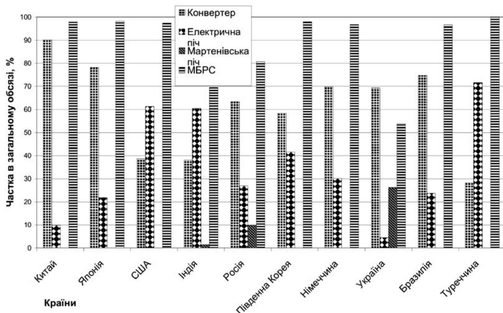
Рис. 1. Технологічна структура виробництва сталі у 2010 році, %.
