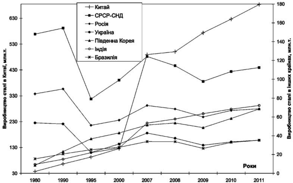
Рис. 2. Динаміка виробництва сталі в країнах перехідної економіки та таких, що розвиваються, в 1980-2011рр. (WSA).
