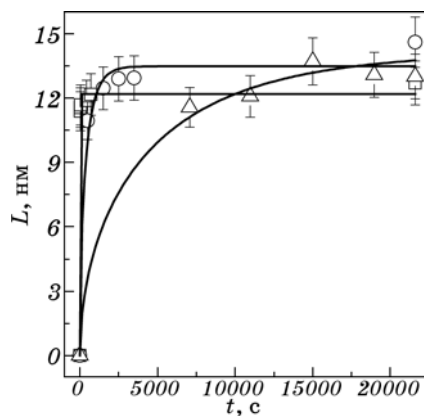
Рис. 3. Зависимость размеров нанокристаллов алюминия от времени для различных температур отжига: \Delta — 460 К, \circ — 501 К, \square — 536 К; сплошные линии — результат расчета по уравнению (4).
