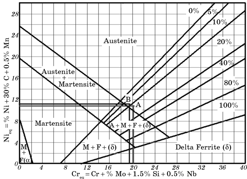
Fig. 1. Schaeffler diagram.
