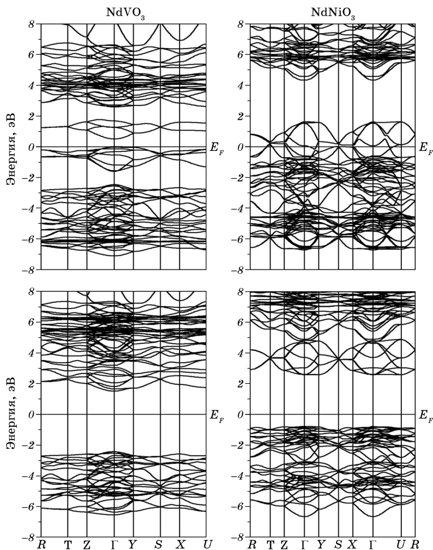
Рис. 3. Дисперсионные зависимости E(\mathbf{k}) вдоль прямых, соединяющих точки высокой симметрии в обратном пространстве зоны Бриллюэна. Верхняя часть рисунка — спин вверх, нижняя — спин вниз, E_F — энергия Ферми.
