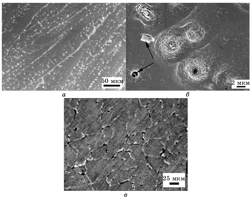
Рис. 3. Микроструктура приповерхностной 3 ( a, б ) и придонной 1 зон ( в ) сплавов Al_xFeCoNiCuCr ( A_1 и A_3 ): глобулярные частицы расположены вдоль границ дендритов ( a ), внутри них ( б ) и по границам зерен ( в ) соответственно.
