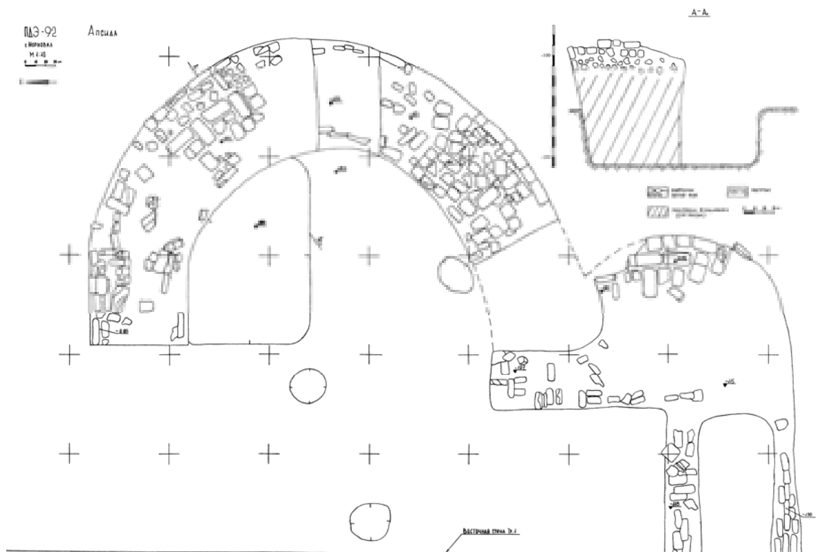
Рис. 12. План кладок апсиди церкви (розкоп 1) і розріз по лінії AA 1 Fig. 12. Plan of masonry of apse of the church (excavation 1) and section of the line AA 1
