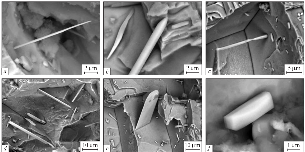
Рис. 2. СЕМ-зображення голчастих (а–с), дощатих (d), пластинчатих (e) та стовбчастих (f) кристалів рабдиту в камаситі на глибокопротравленій поверхні металевого каркаса паласиту Омолон
