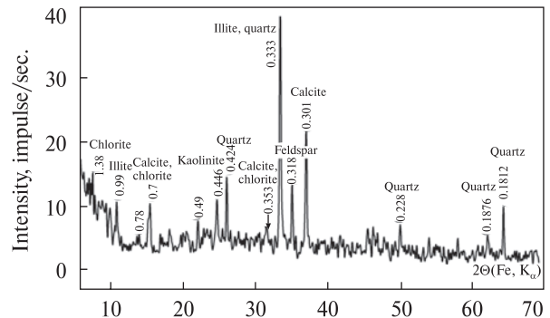
Рис. 4. Фракція <0,01 мм. Склад: гідрослюда, хлорит, каолінит, кварц, кальцит, польовий шпат (плагіоклаз) Fig. 4. Fraction <0.01 mm. Ingredients: illite, chlorite, kaolinite, quartz, calcite, feldspar (plagioclase)
