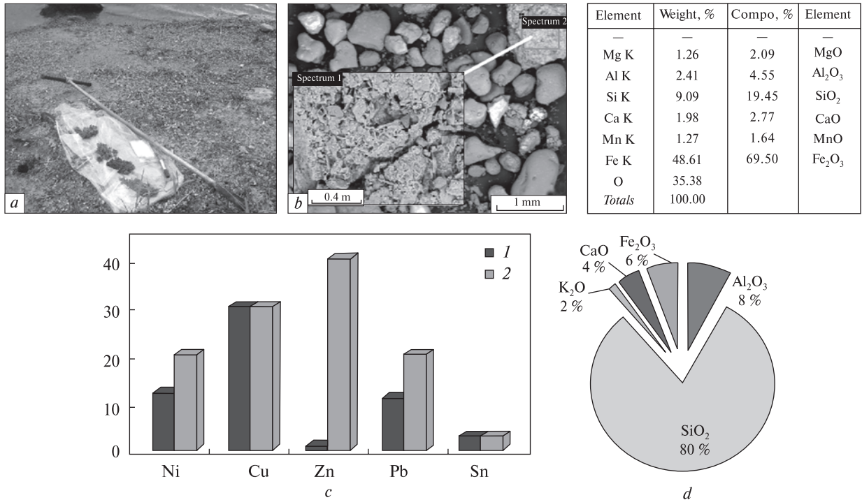
Рис. 2. Зображення: a — процес відбору вертикальної колонки проб у межах берегової смуги Дніпра; b — електронно-мікроскопічний знімок відібраної проби та хімічний склад фрагмента зразка — агрегату з дрібнодисперсних уламкових і глинистих частинок; c — вміст важких металів у складі проби, відібраної у межах прибіжної зони узбережжя Дніпра (1) та регіональне фонове значення (2, [3]), мг/кг; d — розподіл основних компонентів хімічного складу в пробі, відібраної у межах прибіжної зони узбережжя Дніпра
