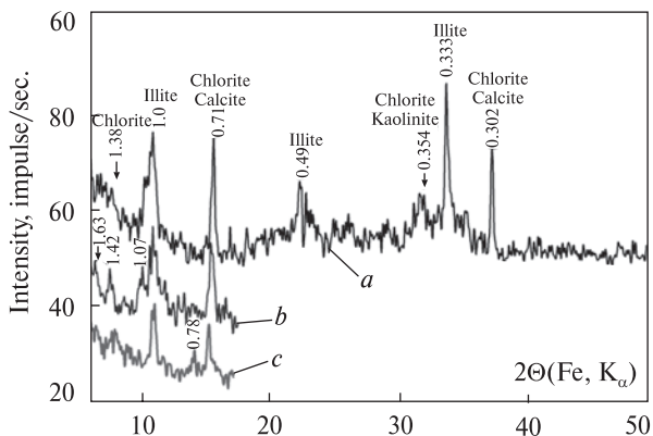
Рис. 3. Фракція <0,001 мм. Склад: гідрослюда, хлорит, каолінит, кальцит, змішаносарувате утворення гідрослюда — монтморилоніт (домішка). a — вихідний, b — насичений етиленгліколем, c — відпалений за T = 550\text{ }^{\circ}\text{C}
