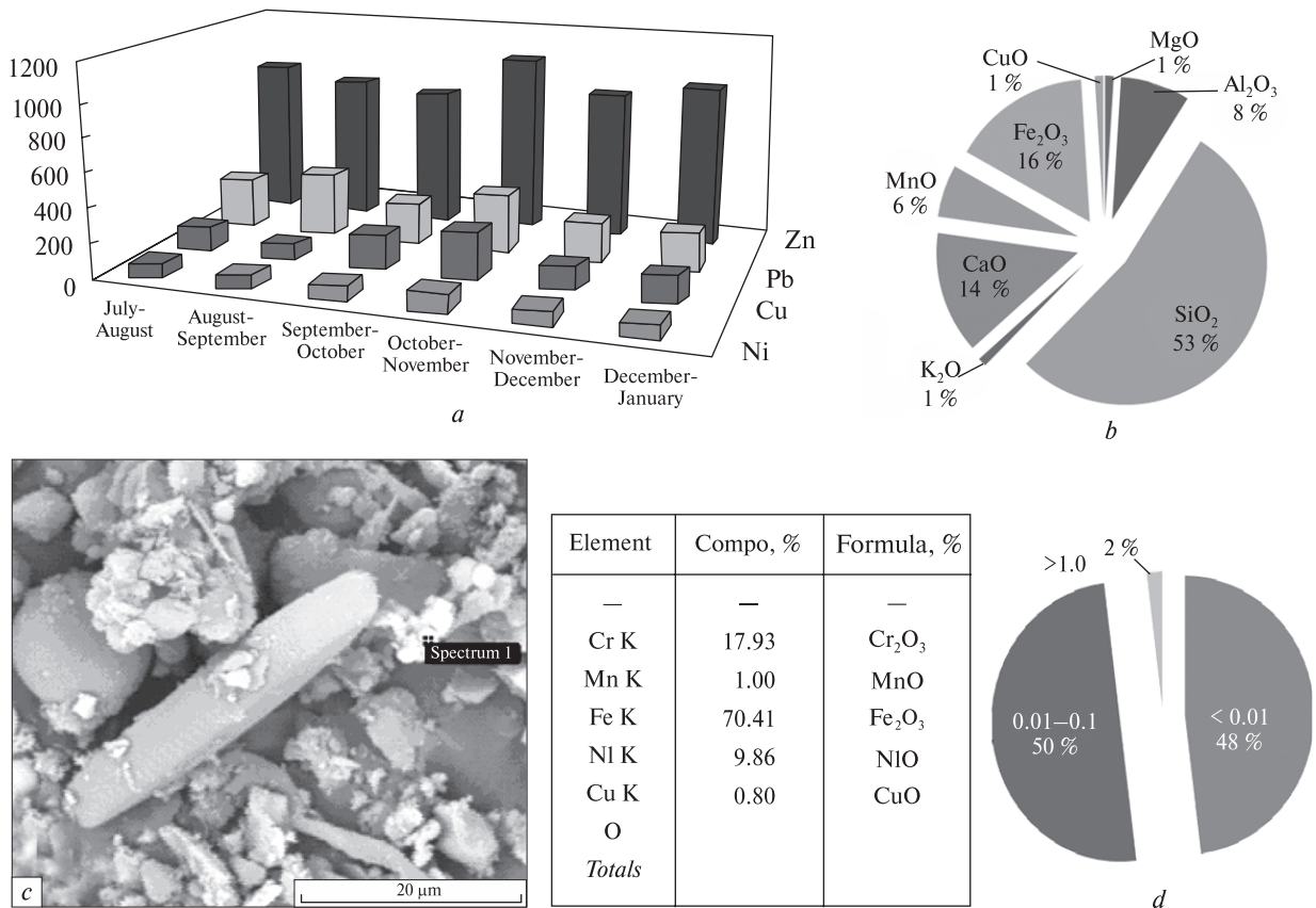
Рис. 8. Характеристики складу річкової завислої речовини: a — розподіл вмісту важких металів у пробах за різні часові інтервали (період з 15 числа попереднього місяця до 15 числа наступного), мг/кг; b — середні показники розподілу основних компонентів хімічного складу в пробах; c — фрагмент електронно-мікроскопічного знімку компонентів речовинного складу зразка, на зображенні представлені сферичні утворення, черепашка фітопланктону, хімічний склад виділеної конкреції свідчить про високий вміст у ній важких металів; d — середні показники розподілу основних гранулометричних фракцій у пробах
