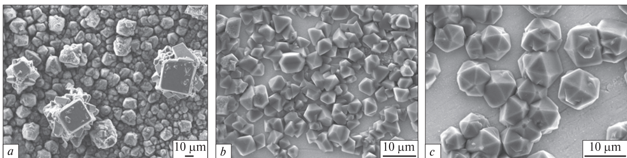
Рис. 1. Загальний вигляд кристалів алмазу на плівці 1: a — центральна частина; b , c — різні крайові частини плівки. Растрові електронно-мікроскопічні знімки (РЕМ знімки; JSM 6700F; LEI; 15,0 кВ; WD 15,0 мм)
