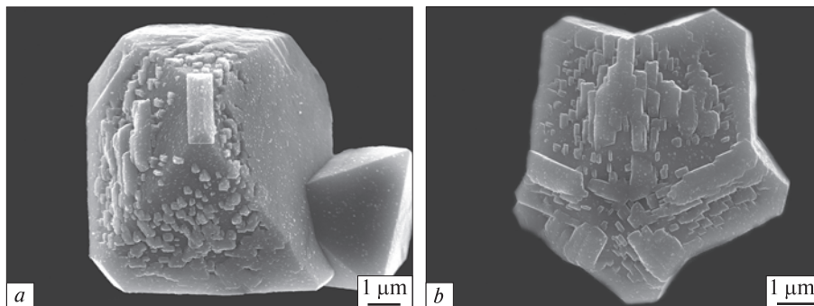
Рис. 7. Кристали алмазу з епітаксійними наростами, плівка 1: a — на октаедрі, b — на зірчастому п'ятиграннику кубо-октаедрів (РЕМ знімки; JSM 6700F; SEI, 15,0 kV; WD — 6,1 мм)
