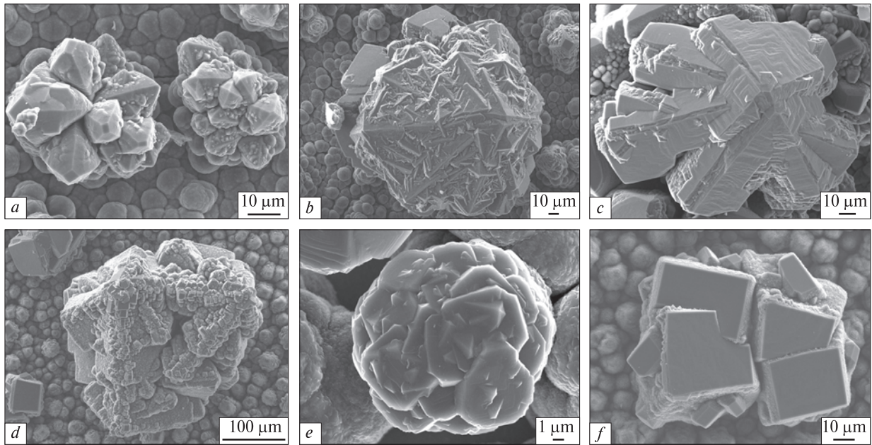
Рис. 4. Агрегати багатогранників алмазу, плівка 2 і плівка 1e: пояснення в тексті (PEM знімки; JSM 6700F; LEI; 15.0 kV; WD, мм: a–d, f – 15,0; e – 9,4)
