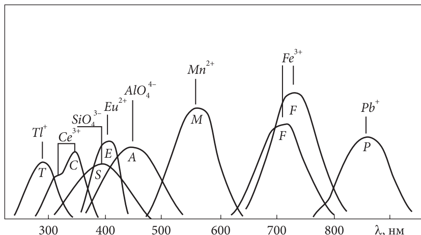
Рис. 9. Основні смуги РЛ-випромінювання у польових шпатах [10]
