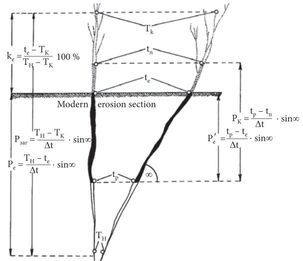
Рис. 2. Принципова схема термобарогеохімічної оцінки розміру вертикального розмаху (у метрах) продуктивного зруденіння P_{\text{зар}} та його найбільш концентрованої частини P_{\text{к}} ; T_H , T_K — температурні характеристики початку і кінця розвитку продуктивної стадії зруденіння; t — вертикальний градієнт температури (°C/100 м), за флюїдними включеннями у мінералах тієї самої стадії; t_p , t_n , t_c — температура гомогенізації включень у мінералах ранніх, пізніх металоносних парагенезисів і розвинутих на рівні сучасного ерозійного зрізу; K_{\text{е}} — коефіцієнт ерозії рудної зони з кутом падіння; P_{\text{с}} і P'_{\text{с}} — розмах зон продуктивного і багатого зруденіння нижче від ерозійного зрізу
