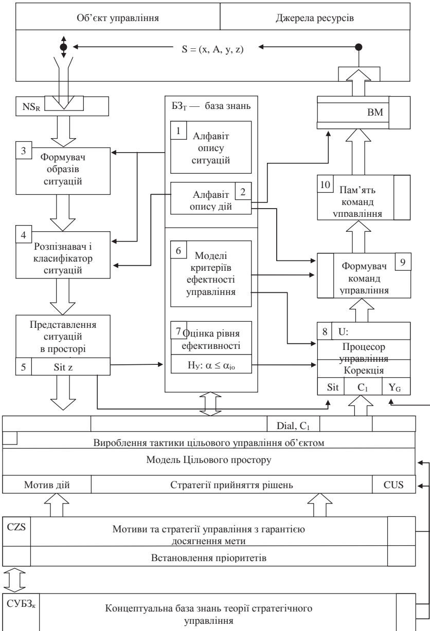
Рис. 2. Модель інформаційних процесів управління діяльністю в інтегрованих системах
