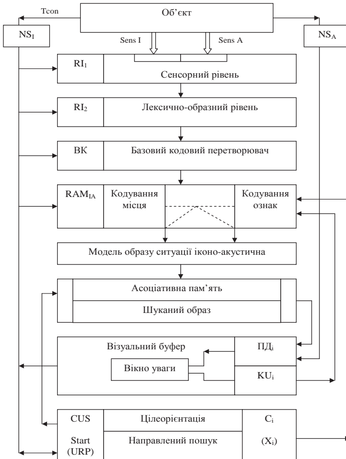
Рис. 4. Структурна схема формування образів ситуацій, де: C_i – цільова координата, (x_i) – потік даних про траєкторію руху, CUS – цілеспрямована система, Strat(URP) – стратегія управління розв'язання проблеми, KU_i – команди управління, ПД_i – потік даних про ситуацію.
