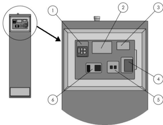
Рис. 2. Візуалізація блоку управління установки: 1 – блок контролю швидкості вентилятора розрідження, 2 – блок живлення 12 В, 3 – блок живлення 5 В, 4 – плата контролера, 5 – блок перетворення температури, 6 – блок-реле включення вентилятора розрідження
