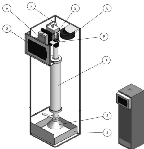
Рис. 1. 3D-модель установки для реалізації авторської технології отримання сорбенту:
