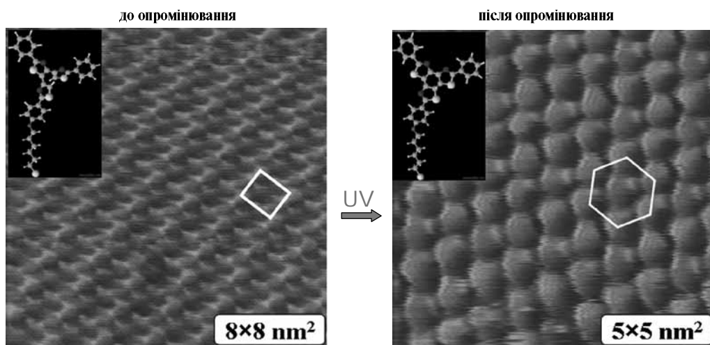
Вплив ультрафіолетового випромінювання на структуру мономолекулярної органічної плівки
