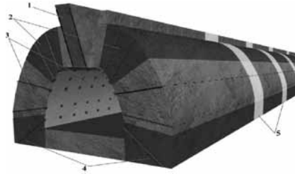
Елементи конструкції АК: 1 – силова та 2 – підпiрні частини, 3 – опори перекриття виробки та 4 – основа конструкції, 5 – запобiжні перемички
