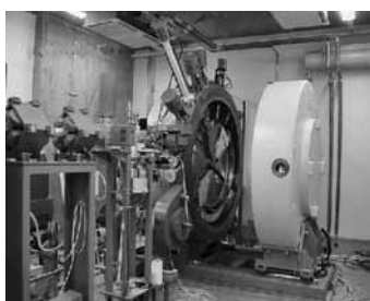
Циклотрон СС-18/9
