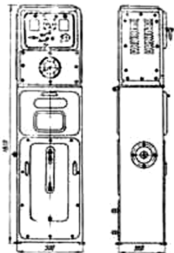
Рис. 2. Ионатор ЛК-25 [12]
