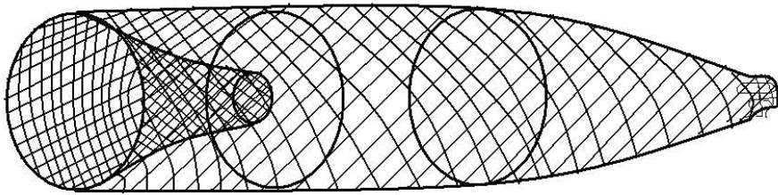
Мал. 4. «Жак одноустенковий» (розмір різний)
