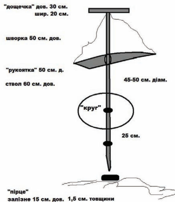
Мал. 5. «Коворота» для свердління дірок у камінцях для «глазків»
