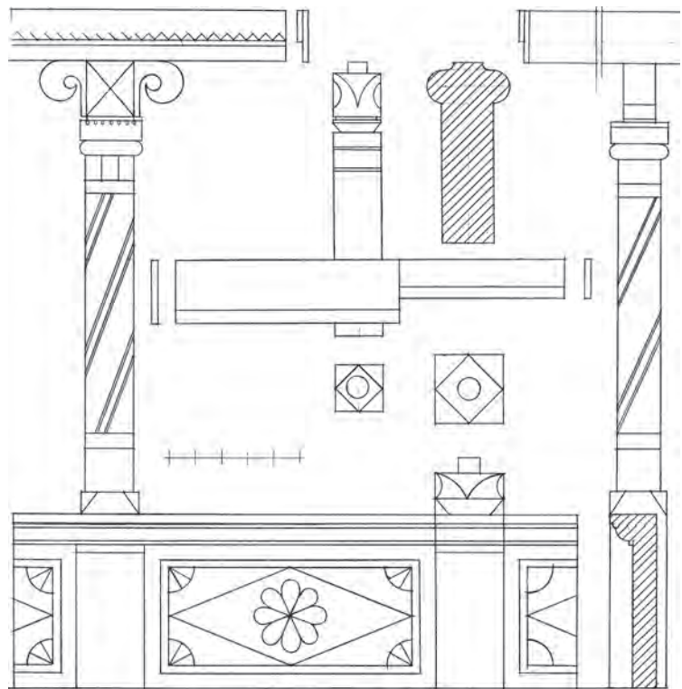
Деталі та конструктивні вузли галереї житлового будинку с. Морюая (Morouaya), Оргеевський р-н. Рис. автора
