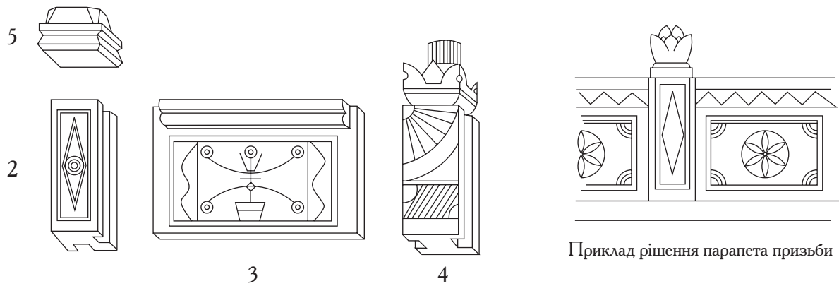
Житловий будинок І. Ротаря в с. Желобок (Zhelobok), Орґеєвський р-н. Фасад. Рисунок автора за матеріалами А. Захарова
