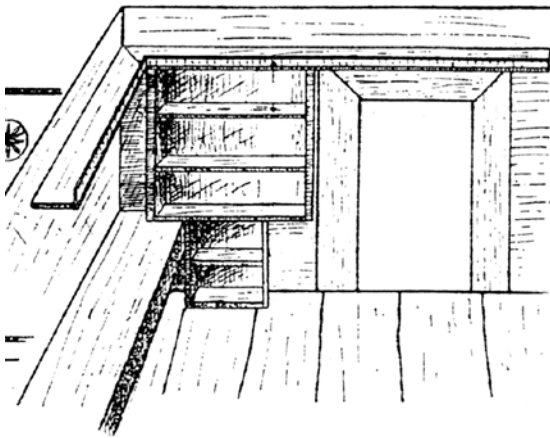
Конструктивне з'єднання нерухокої лави і мисника (Гуцульщина). (За Яном Фальковським)
