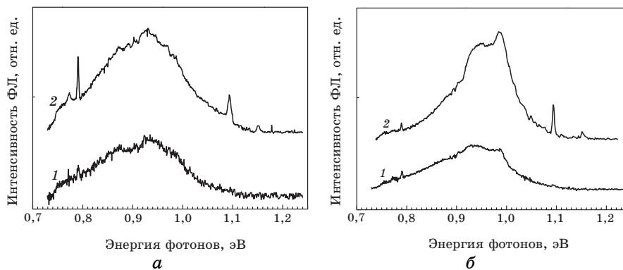
Рис. 3. Снятые при 4,2 \text{ К} спектры ФЛ образцов кремния после имплантации As ( 245 \text{ кэВ} , 4,1 \cdot 10^{16} \text{ см}^{-2} ) и In ( 350 \text{ кэВ} , 3,7 \cdot 10^{16} \text{ см}^{-2} ) при 25^\circ\text{C} ( a ) и 500^\circ\text{C} ( б , кривая 1) и отжига ( 900^\circ\text{C} , 60 мин). a — образец без геттера (кривая 1) и с геттером (кривая 2); кривая 2 на рисунке б — спектр ФЛ образца после «горячей» имплантации As ( 245 \text{ кэВ} , 5 \cdot 10^{16} \text{ см}^{-2} ) и In ( 350 \text{ кэВ} , 4,5 \cdot 10^{16} \text{ см}^{-2} ) и отжига ( 900^\circ\text{C} , 45 мин).
