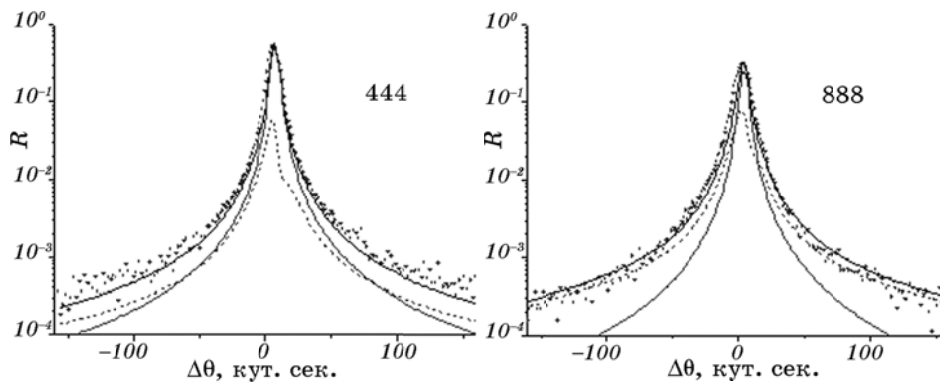
Рис. 8. Виміряні і теоретичні КДВ (відповідно маркери і товсті суцільні лінії) для рефлексів ГГ (444) і (888), випромінення \text{CuK}_{\alpha 1} . Тонкі суцільні та штрихові лінії описують відповідно когерентні компоненти КДВ та внески ДР від кластерів і дислокаційних петель.
