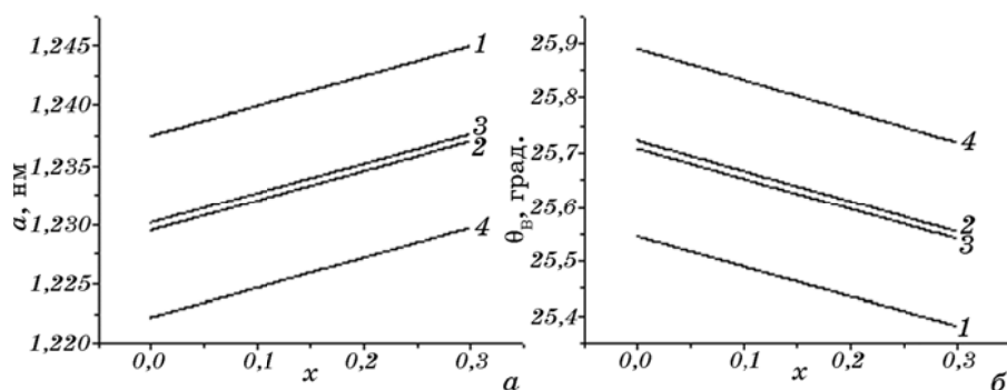
Рис. 2. Залежності сталої ґратниці ( a ) і Брегґового кута ( б ) для рефлексу ГГГ (444), випромінення \text{CuK}_{\alpha 1} , від концентрації антиструктурних дефектів \text{Gd}^{3+} в октаедричних позиціях ( x ) при різних концентраціях антиструктурних дефектів \text{Gd}^{3+} у додекаедричних позиціях ( y ) і вакансій \text{Gd}^{3+} в октаедричних позиціях ( z ): 1 — y = 0; z = 0 ; 2 — y = 0,1; z = 0 ; 3 — y = 0; z = 0,1 ; 4 — y = 0,1; z = 0,1 .
