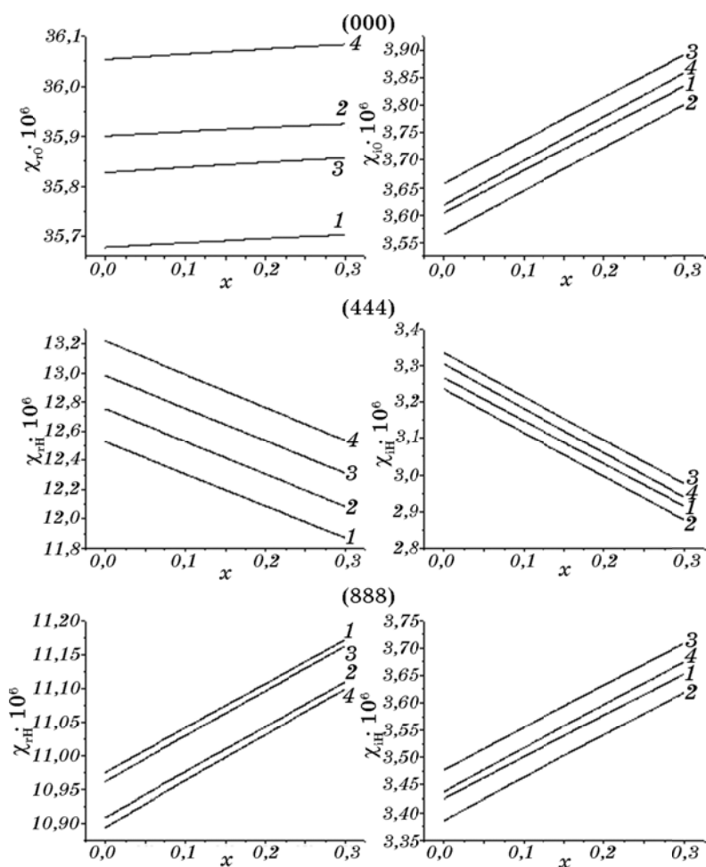
Рис. 3. Залежності дифракційних параметрів кристалу гранату ГГГ для рефлексів (000), (444) і (888), випромінювання \text{CuK}\alpha_1 , від концентрації антиструктурних дефектів \text{Gd}^{3+} в октаедричних позиціях ( x ) при різних концентраціях антиструктурних дефектів \text{Gd}^{3+} у додекаедричних позиціях ( y ) і вакансій \text{Gd}^{3+} в октаедричних позиціях ( z ): 1 — y=0 ; z=0 ; 2 — y=0,1 ; z=0 ; 3 — y=0 ; z=0,1 ; 4 — y=0,1 ; z=0,1 .
