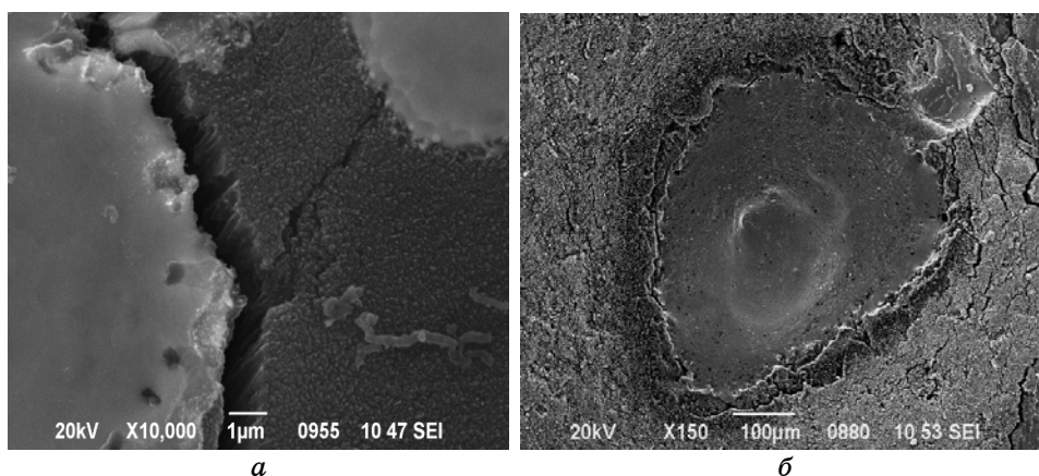
Рис. 3. Электронно-микроскопический снимок катода УНТ на Ni: a — до лазерного облучения; б — после лазерного облучения.
