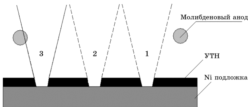
Рис. 2. Схема переноса УНТ с Ni-подложки (катод) на Мо-проволоку (анод) под воздействием лазерного излучения, поясняющая смену направления эмиссионного тока.
