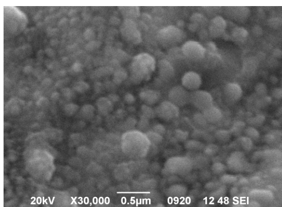
Рис. 4. Электронно-микроскопический снимок наноструктурной пленки на Mo-аноде.
