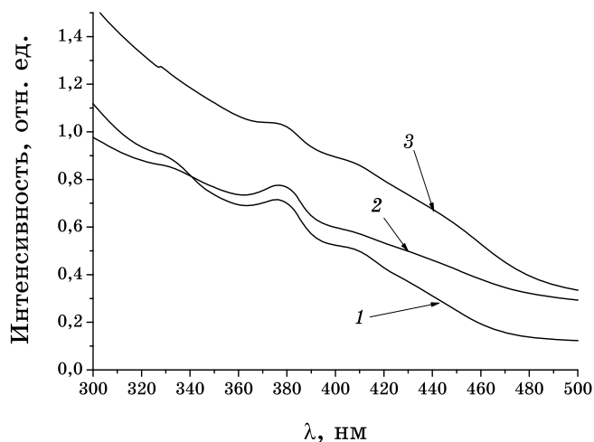
Рис. 3. Спектры поглощения мезоморфных стекловидных нанокомпозитов в системах \text{Cd}, M | \text{C}_5\text{H}_{11}\text{COO} (эквимольного состава), допированных наночастицами сульфида кадмия (содержание CdS — 1 мол.%): 1 — M = \text{Li}^+ , 2 — \text{Na}^+ , 3 — \text{K}^+ .
