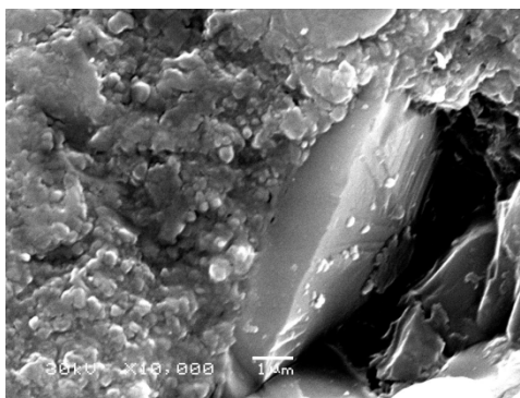
Рис. 2. СЭМ-изображение во вторичных электронах поверхности излома тонкозернистого вещества со сложным многоуровневым глобулярным строением силикатных минералов в метеорите Крымка. На грани крупного кристалла оливина (справа) расположены нанокристаллы хромита (белое) метаморфического происхождения.
