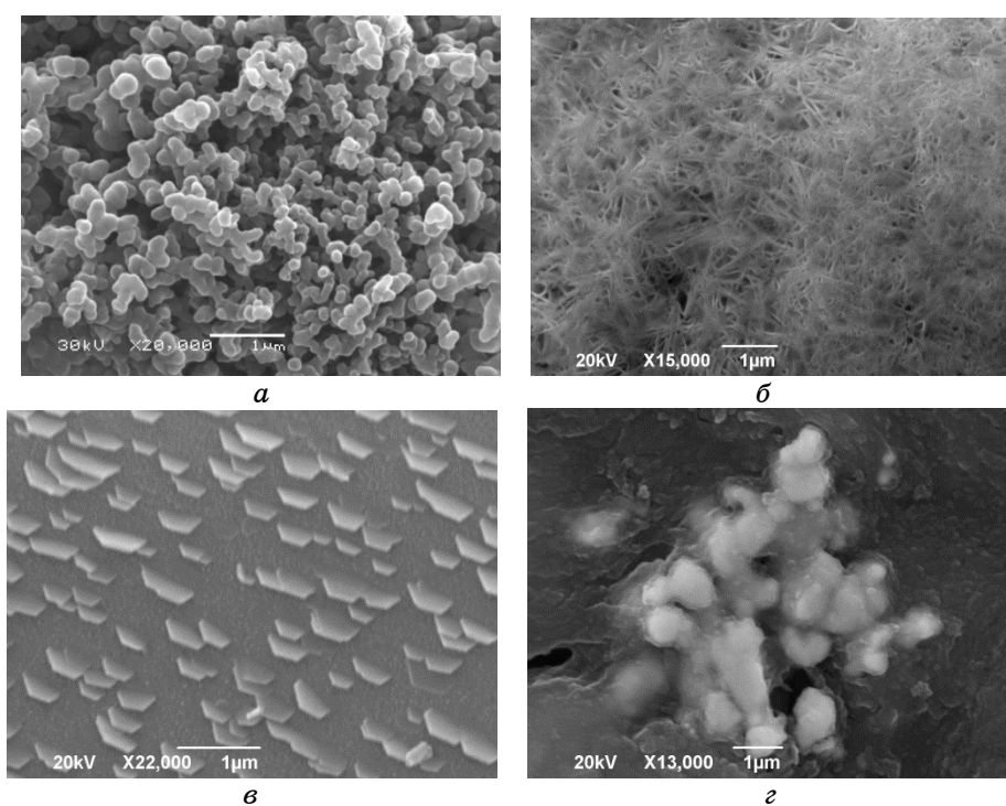
Рис. 6. СЭМ-изображение во вторичных электронах продуктов земного выветривания в метеоритах: а) сотовидные агрегаты глобул гидроксидов железа, развитые на поверхности скола углистого хондрита Allende; б) скопленные игольчатых кристаллов гетита на полированной поверхности хондрита Крымка; в) гексагональные пластинки гематита (?), расположенные закономерно на поверхности силикатного зерна из палласита Омолон; г) многоуровневое глобулярное строение агрегата самородного серебра, которое ассоциирует с Fe, Ni, S-гидроксидами в хондрите Крымка.
