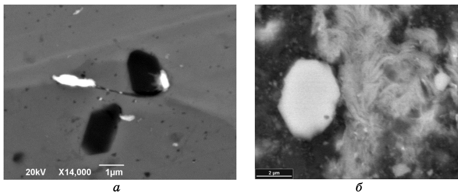
Рис. 5. СЭМ-изображение в отраженных электронах метаморфогенных минералов в полированных шлифах метеорита Крымка: а ) уникальные включения самородного вольфрама (белое) в металлическом шарике (серое) одной из хондр (нанозерна вольфрама расположены по трещинам и межфазовым границам, темно-серые пятна — вероятно фосфиды, черное — кристаллы хромита); б ) агрегат тончайших нитей филлосиликатов (светло-серые), белое — кристалл магнетита, темно-серое — силикаты.
