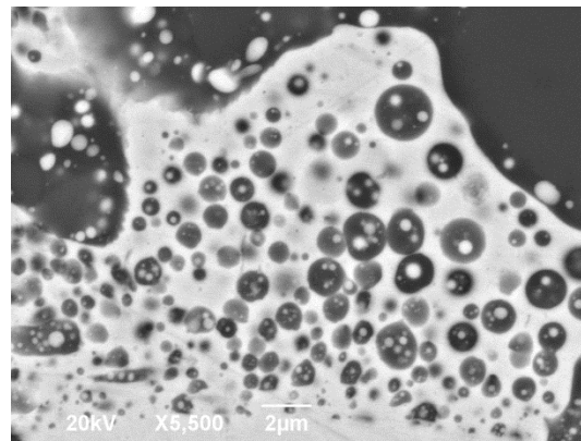
Рис. 4. СЭМ-изображение в отраженных электронах сложной лиофильной эмульсии тенита (белое) и силикатов, образованной в результате ударного плавления в хондрите Княгиня.
