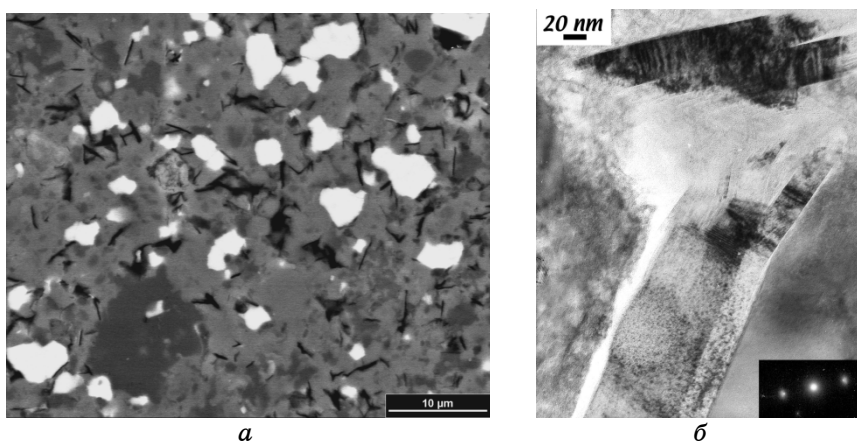
Рис. 3. Кристаллы графита в углистых ксенолитах хондрита Крымка: а) СЭМ-изображение в отраженных электронах кристаллов графита (черное), которые расположены по межфазовым границам зерен (белое — троилит, серое — силикаты); б) трансмиссионное ЭМ-фото кристалла графита. Четкие пятна на электронно-дифракционном изображении указывают на кристаллическое строение графита. ТЭМ-исследование выполнено И. Вебер (Ин-т планетологии, Мюнстер, ФРГ) [8].
