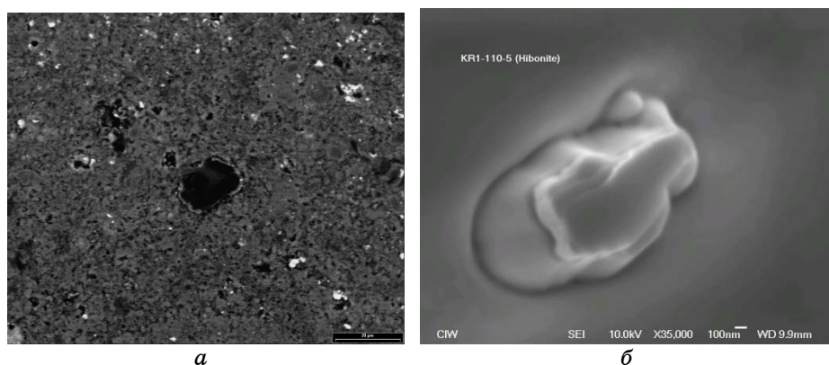
Рис. 1. Сканирующее электронно-микроскопическое (СЭМ) изображение гибонита из метеорита Крымка: а ) зерно (черное), расположенное в силикатном веществе углистого ксенолита ВК-13 (полированный шлиф, отраженные электроны); б ) досолнечное зерно, выделенное химическим методом из метеорита и расположенное на золотой пластинке. Фото для статьи любезно предоставлено Л. Ниттлером (Ин-т Карнеги, Вашингтон, США).
