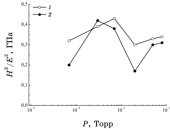
Рис. 6. Міцність ( H^3/E^2 ) покриттів TiAlSiN від тиску азоту: 1 — після осадження; 2 — після вакуумного відпалу.
