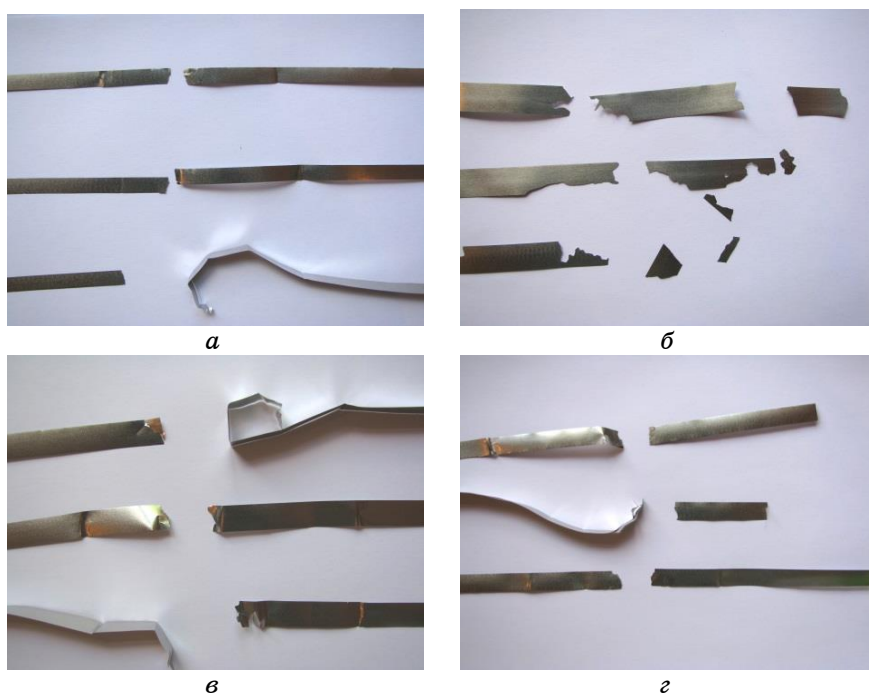
Рис. 1. Внешний вид разрушенных образцов: a — NHRS-(Co-1) шириной 6,5 мм; б — NHRS-Co-2; в — NHRS-(Co-1) шириной 10 мм; г — NHRS-(Co-2).
