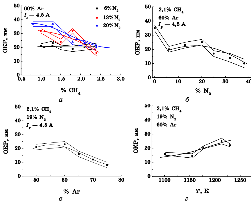
Рис. 6. Зависимость размера ОКР наноструктурных алмазных плёнок, синтезированных из газовой смеси \text{CH}_4/\text{H}_2/\text{Ar}/\text{N}_2 , от: а) концентрации метана, б) концентрации азота, в) концентрации аргона, з) температуры синтеза.
