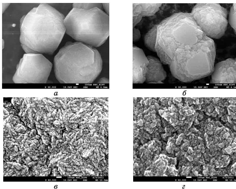
Рис. 2. Микроструктура поверхности алмазных покрытий, полученных из газовой смеси \text{CH}_4/\text{H}_2/\text{Ar}/\text{N}_2 с содержанием аргона 60% и разным содержанием остальных компонентов газовой фазы: верхний ряд — концентрация метана 0,8%, концентрация азота — а) 6%, б) 19%; нижний ряд — концентрация метана 1,5%, концентрация азота — в) 6%, г) 19%.
