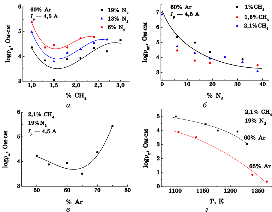
Рис. 7. Зависимость величины удельного сопротивления наноструктурных алмазных покрытий, синтезированных из газовой смеси CH 4 /H 2 /Ar/N 2 : а) от концентрации азота, б) от концентрации метана, в) от концентрации аргона, г) от температуры синтеза.
