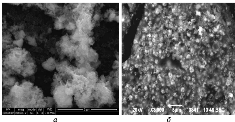
Рис. 2. Електронні фотографії кремнезему ( a ) та гідрозолю ( б ), модифікованого йодидом міді. Концентрація \text{CuI} — 37,5% (мас.).
