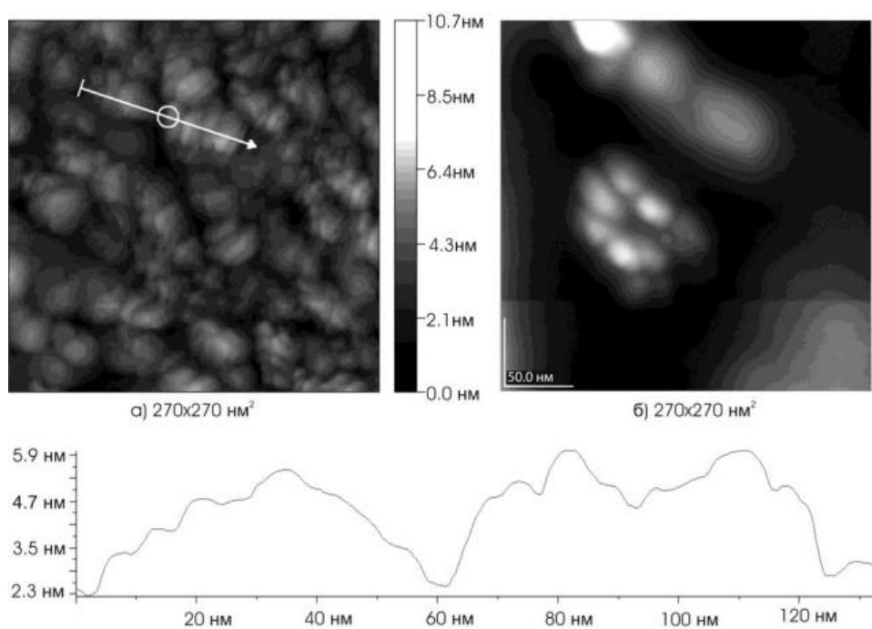
Рис. 1. (а) СТМ-снимок поверхности кремния Si(111) после напыления золота 5 мин (профиль внизу соответствует стрелке); (б) снимок АСМ наночастиц золота на поверхности кремния.
