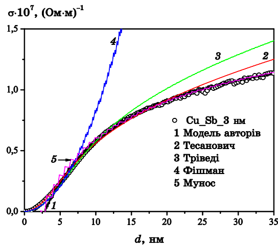
Рис. 4. Розмірні залежності питомої провідності свіжнанесеної на підшар сурми товщиною 1 нм плівки міді (квадрати — експериментальні дані) при T = 78 К; суцільні криві — теоретична апроксимація моделями [8] (1), [3] (2), [4] (3), [5] (4), [7] (5).
