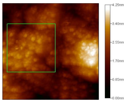
Рис. 7. СТМ-изображение поверхности АМС \text{Fe}_{82}\text{Si}_4\text{B}_{14} при температуре 700^\circ\text{C} ( 54,0 \times 54,0 нм).
