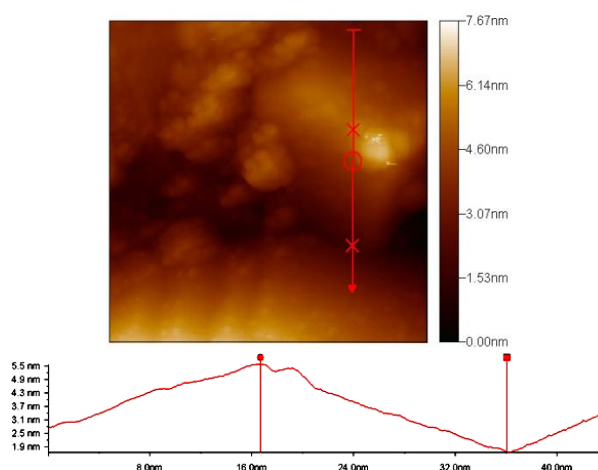
Рис. 4. СТМ-изображение поверхности АМС \text{Fe}_{82}\text{Si}_4\text{B}_{14} при температуре 500^\circ\text{C} ( 54,0 \times 54,0 нм).
