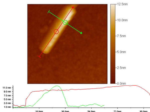
Рис. 5. Наностержни на поверхности АМС \text{Fe}_{82}\text{Si}_4\text{B}_{14} при T = 500^\circ\text{C} ( 126 \times 126 нм).
