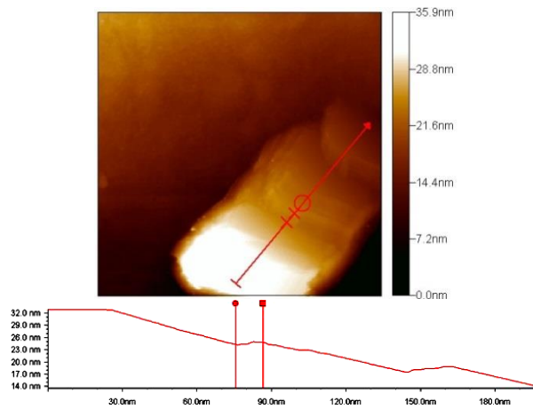
Рис. 8. СТМ-изображение формирования нанорельефа на поверхности АМС \text{Fe}_{82}\text{Si}_4\text{B}_{14} при температуре 700^\circ\text{C} ( 270 \times 270 нм).
