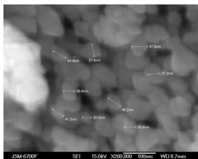
Рис. 4. SEM-зображення синтезованого матеріалу, якого відпалено при 873 К.
