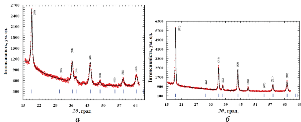
Рис. 2. Дифрактограми зразка LiMn _{1,95} Fe _{0,05} O _4 за температури відпалу у 873 К (а) та 1073 К (б).
