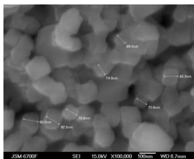
Рис. 5. SEM-зображення синтезованого матеріалу, якого відпалено при 1073 К.
