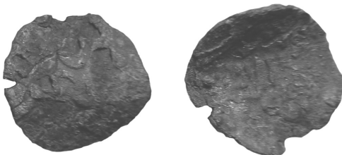
Рис. 11 (а, б) Золотоординський мідний пул
