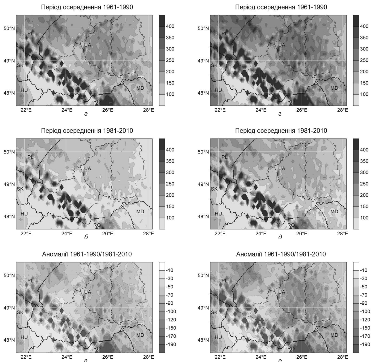
Рис. 7. Оцінки середньої багаторічної питомої потужності вітру та її аномалії на висоті 30 м (а, б, в) та 50 м (г, д, е) з використанням логарифмічного профілю вітру ( Вт \cdot м^{-2} )
