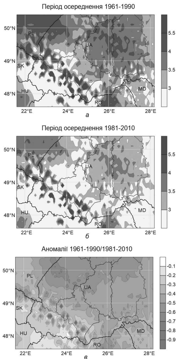
Рис. 1. Середня багаторічна швидкість вітру та її аномалії ( m \cdot c^{-1} )
