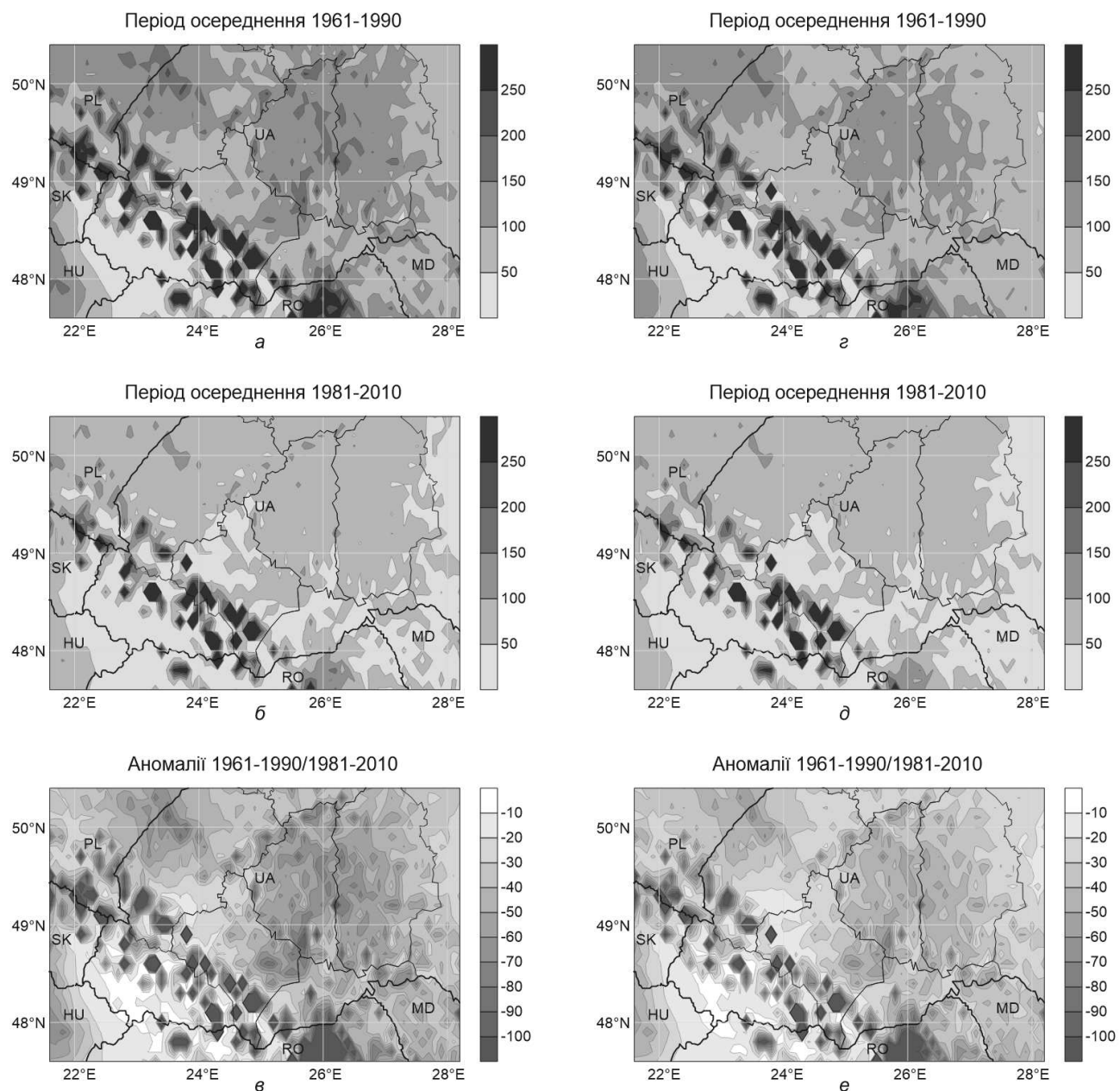
Рис. 6. Оцінки середньої багаторічної питомої потужності вітру на висоті 10 м з урахуванням отриманих поправок методом I (а, б), методом II (с, д) та їх аномалії (в, е) ( Вт \cdot м^{-2} )
