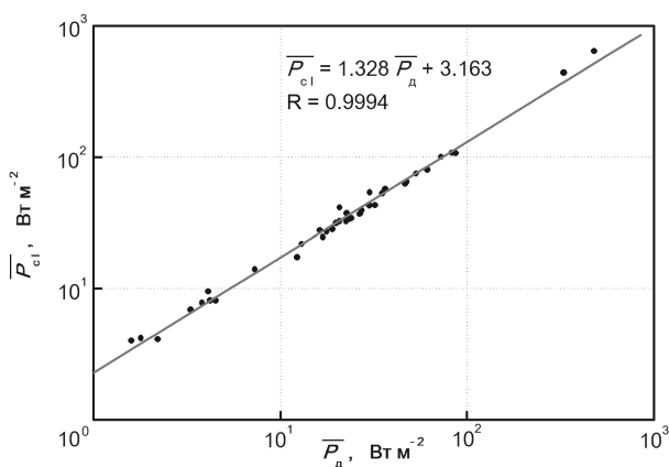
Рис 5. Залежність між багаторічними середніми значеннями питомої потужності вітру розрахованими на основі строкових ( P_{cI} ) та середніх добових ( P_d ) значень швидкості вітру (період осереднення 1981-2010 рр.)
