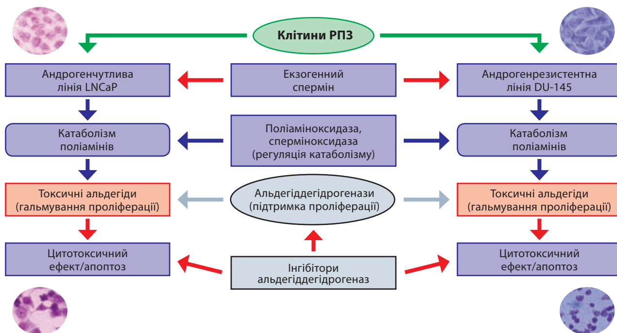
Рис. 4. Схема загального механізму виникнення тандемного альдегідного шоку , викликаного поєднаним впливом Spn і інгібіторів ALDH на клітини РПЗ
