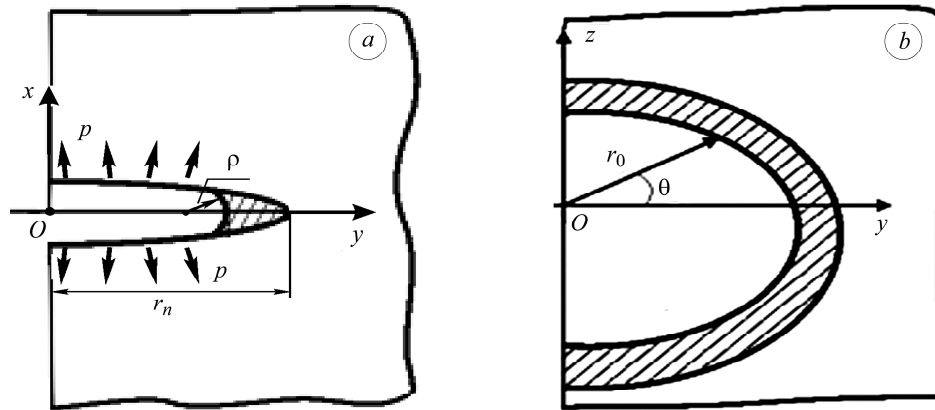
Рис. 4. Схема перерізу безмежного тіла зі сплюсненою мікропорожниною координатними площинами xOy (а) та zOy (б).
