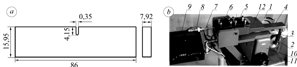
Рис. 6. Схематичне зображення зразка для випробувань (а) та загальний вигляд установки (б): 1 – електродвигун; 2 – ексцентрик; 3 – шатун; 4 – важіль; 5 – рухомий захоп; 6 – нерухомий захоп; 7 – хвилевід сигналів акустичної емісії; 8 – первинний перетворювач акустичної емісії; 9 – вимірювальний модуль; 10 – стійка; 11 – станина; 12 – кожух тензометричного вимірювального мосту.
