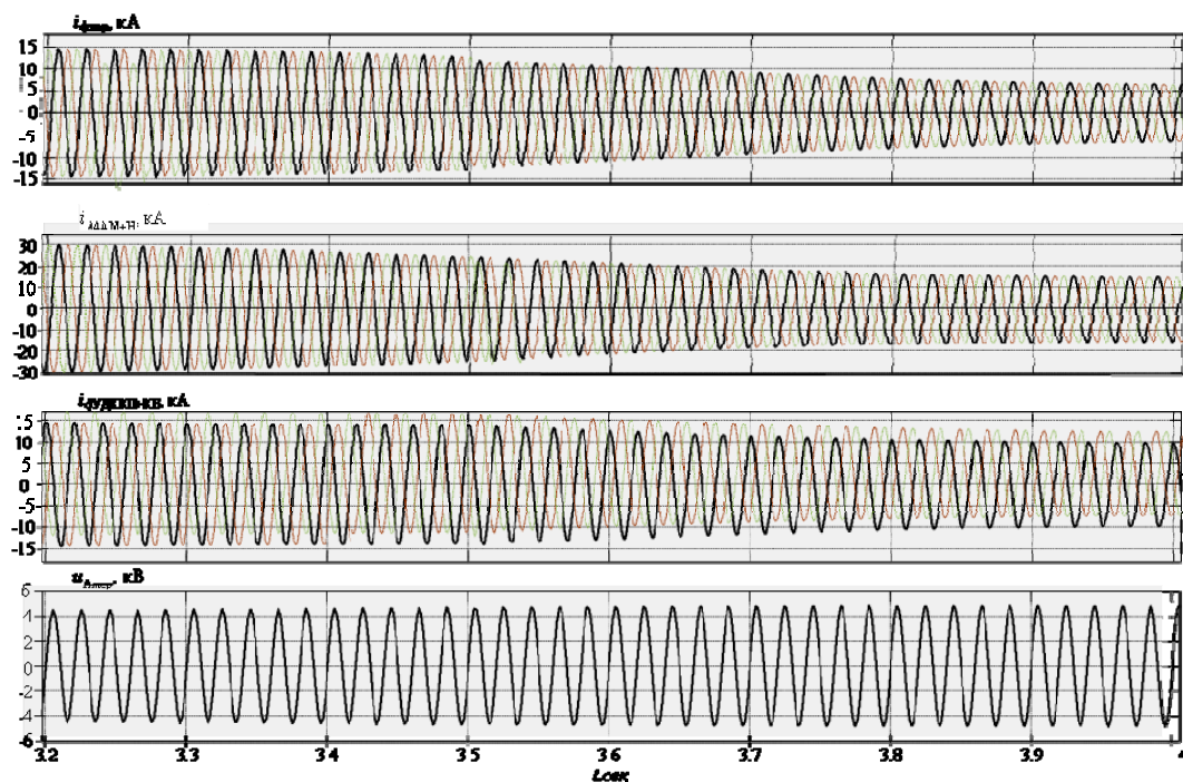
Рис. 3. Фрагмент часової діаграми з відображенням найбільш суттєвих змінень монотонно спадаючих перехідних пускових струмів і монотонно зростаючої напруги у процесі встановлення усталеного режиму
