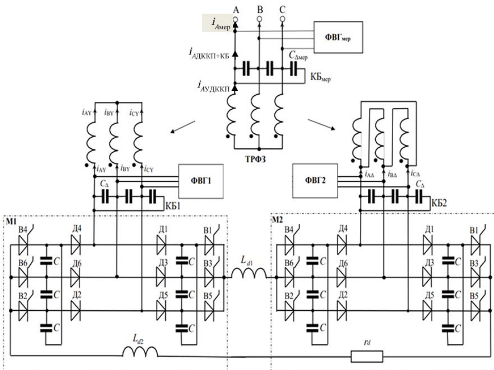
Рис. 1. Модель мережі з УДККП
