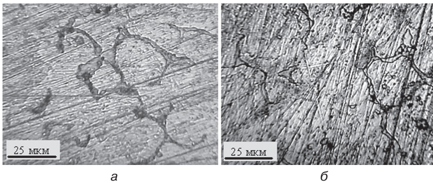
Рис. 4. Междеренные пространства в сплаве № 2, V = 0,20 Тл: скорость охлаждения, °С/с: а – 25, б – 50
