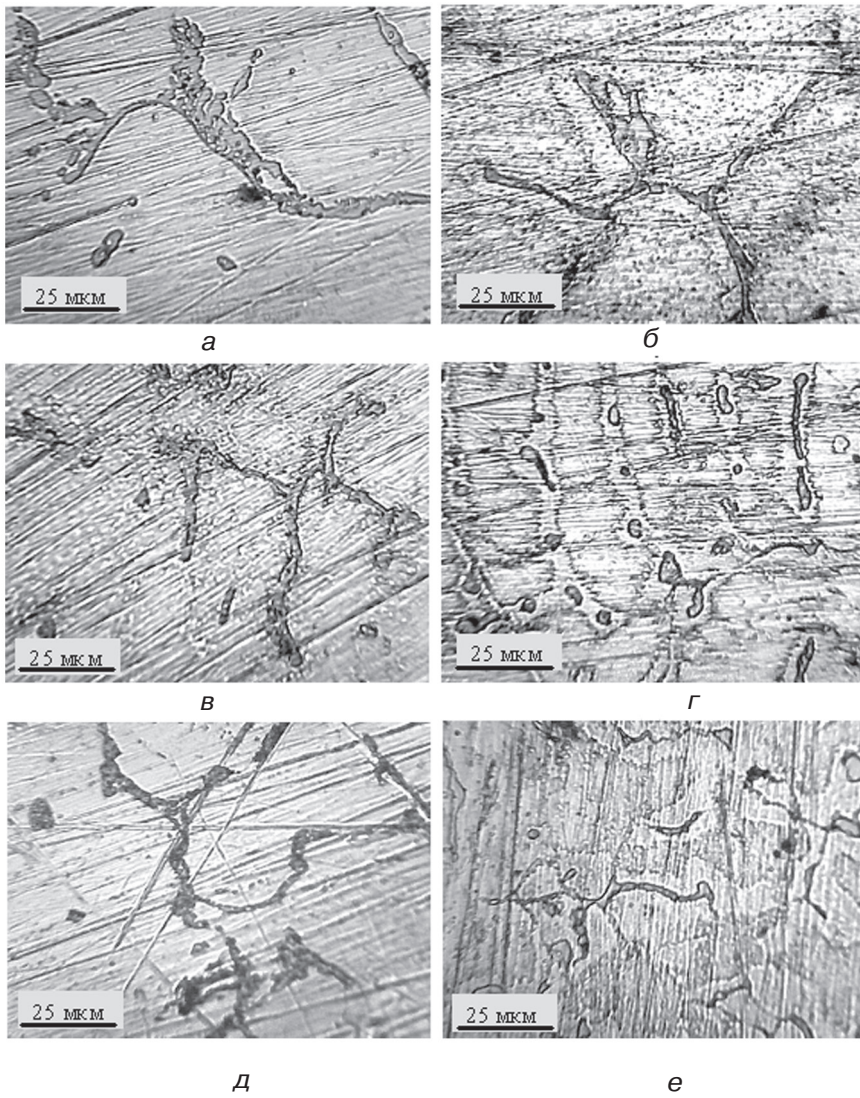
Рис. 3. Междеренные пространства в сплаве № 2: а, в, д – V = 0 Тл; б, г, е – 0,10 Тл; скорость охлаждения, °С/с: а, б – 10; в, г – 25; д, е – 50
