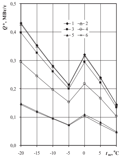
Рис. 2. Залежність питомої теплопродуктивності Q^* повітрянагрівача від температури навколишнього середовища t_{\text{нс}} при застосуванні різних поверхонь теплообміну: 1-4 – пакети пластин із нанокompозитів ( \lambda = 30, 5, 1, 0,2 \text{ Вт/(м}\cdot\text{К)} ); 5, 6 – пакети пластин та пучки труб з КТП із нержавіючої сталі ( \lambda = 30 \text{ Вт/(м}\cdot\text{К)} ).
