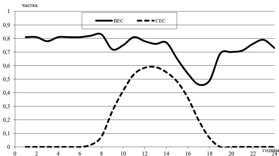
Рис. 1. Фактичні профілі навантаження ВЕС та СЕС в ОЕС України протягом доби 13 жовтня 2018 р.
