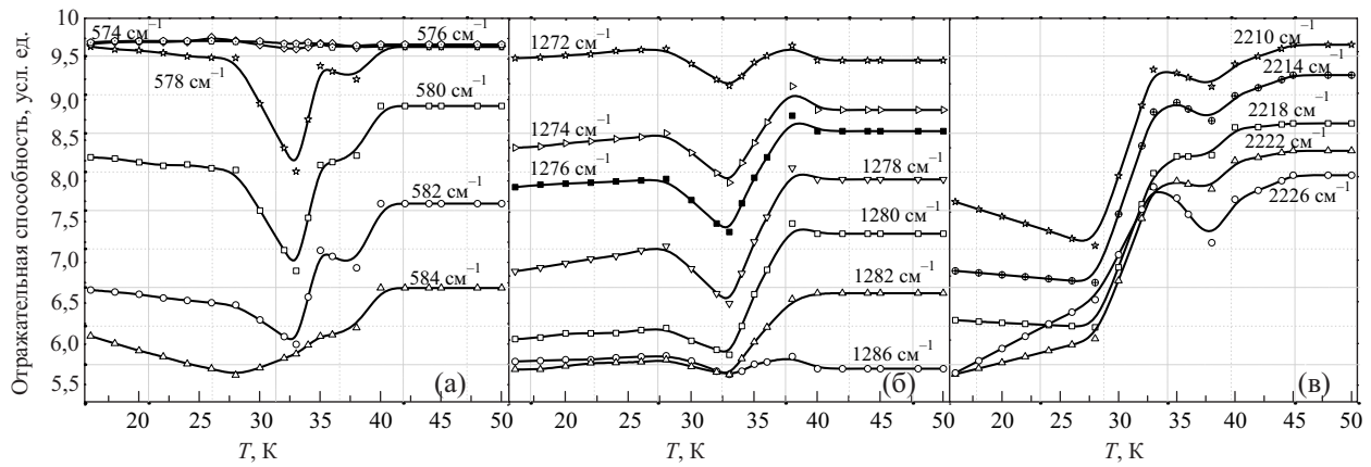
Рис. 5. Термостимулированные изменения положения низкочастотной границы полосы поглощения молекулы закиси азота: деформационные (а); продольные асимметричные (б) и продольные симметричные колебания (в). Кривые смещены по оси Y.
