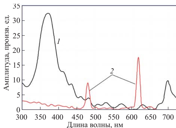
Рис. 2. Характерный спектр криоконденсационного излучения (кривая 1) [9]. Кривая 2 — опорный сигнал калибровочных фильтров.
