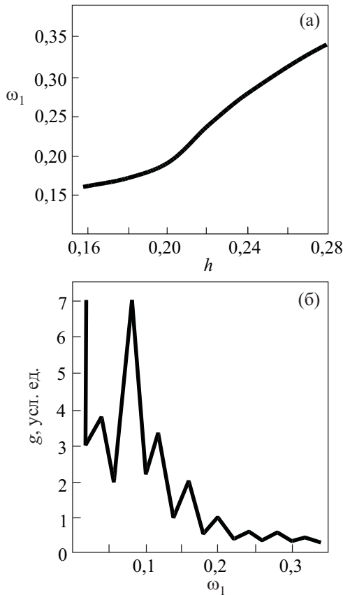
Рис. 4. Зависимость основной частоты нутации \omega_1 от амплитуды внешнего поля h при \varepsilon = 0,3 и \gamma = 0,05 (а) и плотность частот нутации моментов g при \varepsilon = 0,4 , \gamma = 0,05 и h = 0,24 (б).
